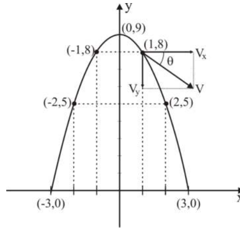
Şekil 10.1. y=9-t^2 parabolü
