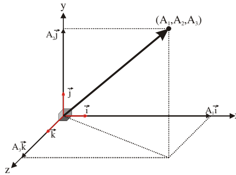
Şekil 6.8. Bir Vektörün Bileşenleri
