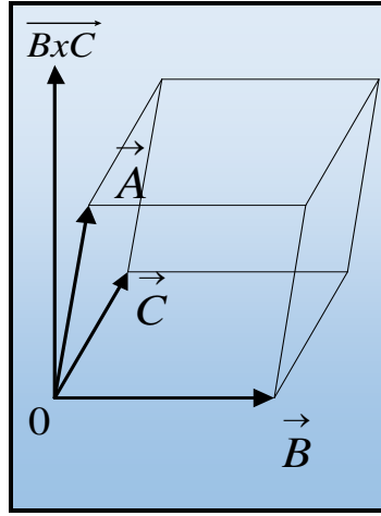
Şekil 6.13. \vec{A}, \vec{B}, \vec{C} üzerine kurulan paralelyüzlünün hacmi
