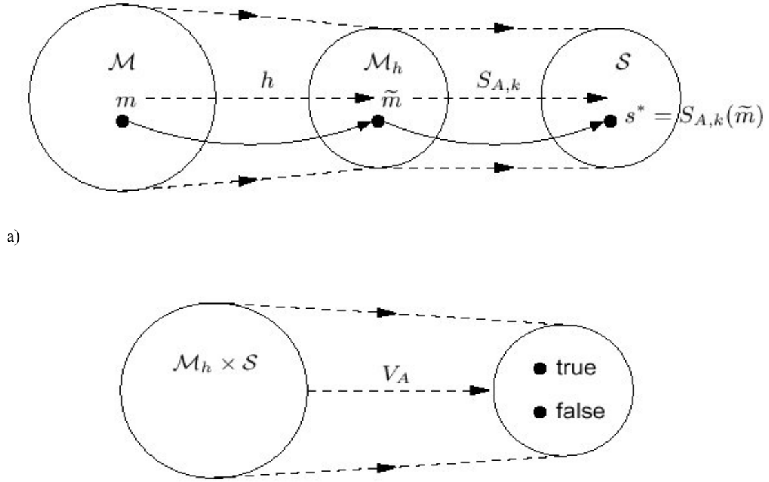
Şekil.5.2. ilaveli bir dijital imza projesinin şeması
