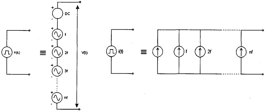
Şekil 4.2: Periyodik gerilim ve akım kaynağının FOURIER dönüşümü
