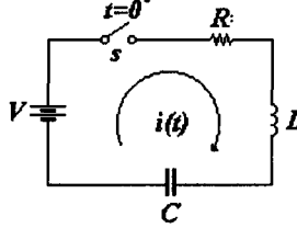
Şekil 5.1: Seri RLC
