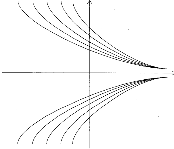
Şekil 1.2: y'=-y 'nin çözüm eğrileri ve eğim alanı.
