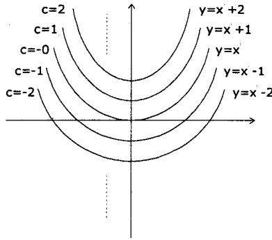
Şekil 1.1: y = x^2 + c genel çözümüne ait grafik (Parabol ailesi)
