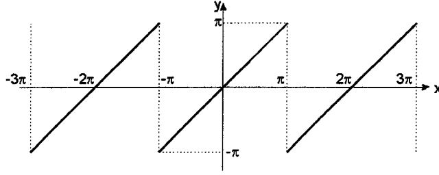
Şekil 4.1: f(x)=x fonksiyonunun 2\pi periyodlu grafiği.
