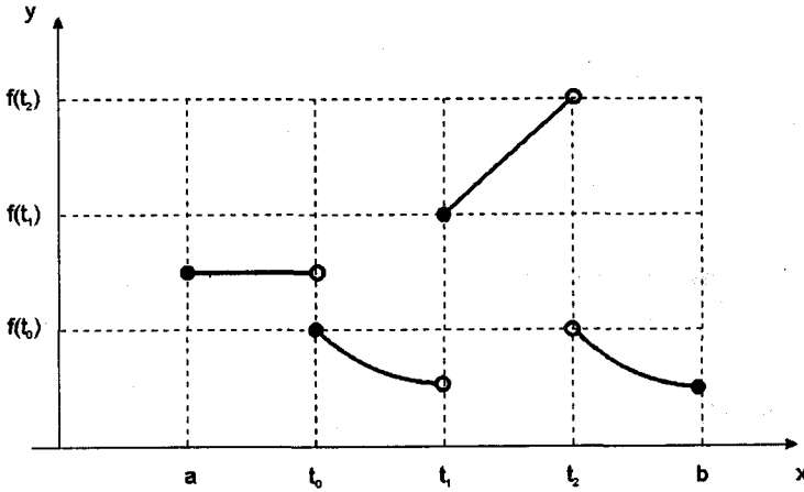
Şekil 3.1: Parçalı sürekli bir fonksiyonda sıçrama değerleri
