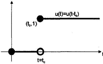
Şekil 3.3: t=t_0 noktasında u(t) birim basamak fonksiyonunun sıçraması
