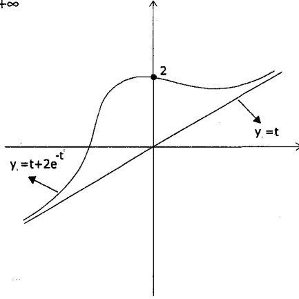
Şekil.1.3. y_1(t) = t + 2e^{-t^2} , y_2(t) = t eğrileri.
