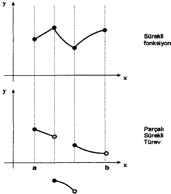
Şekil 3.4. f' 'nin f 'in grafiğine göre süreksizlik grafiği
