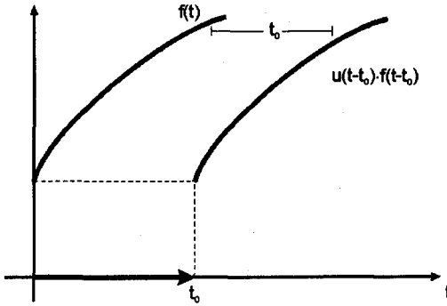
Şekil 3.5: f(t) 'nin t_0 birim sağa kaydırılması.
