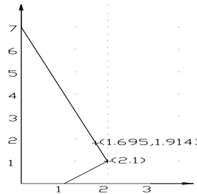
Şekil.7. Problemin yeni aşıkâr çözümü
