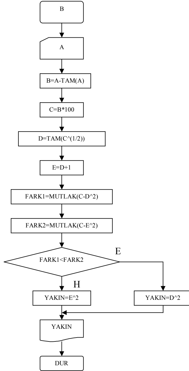
Şekil 4.5.17. Ondalık kısmı iki haneli girilen bir rasyonel sayının ondalık kısmının sayı değerinin en yakın tam kare sayıya uzaklığını bulan akış şeması.
