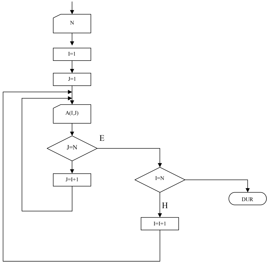
Şekil 4.7.1. NxN' lik bir matrisin girişini yapan akış şeması
