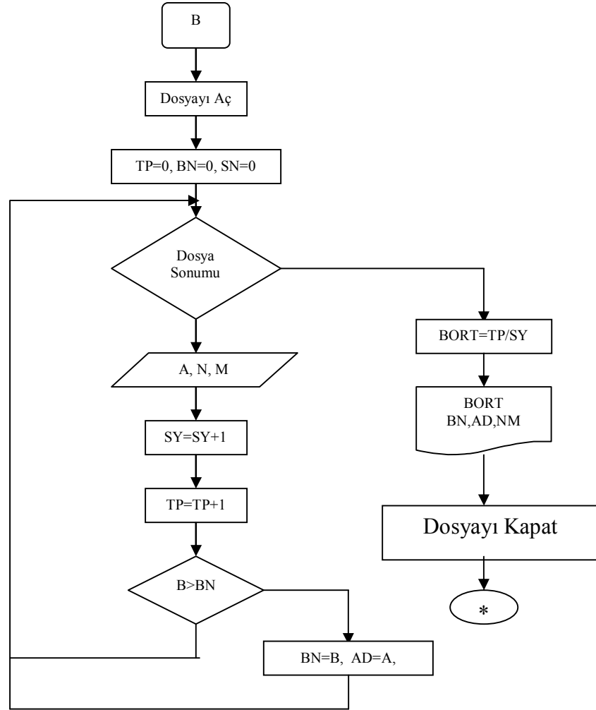
Şekil 5.2.8: Sırasal erişimli bir dosyadan sınıf ortalamasının ve en başarılı öğrencinin bulunmasına ilişkin akış şeması
