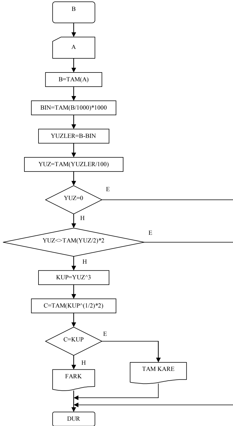
Şekil 4.5.15. Girilen bir rasyonel sayının tam kısmının yüzler hanesindeki değeri çift ise bu değerin küpünün bir tam kare olup olmadığını bulan akış şeması
