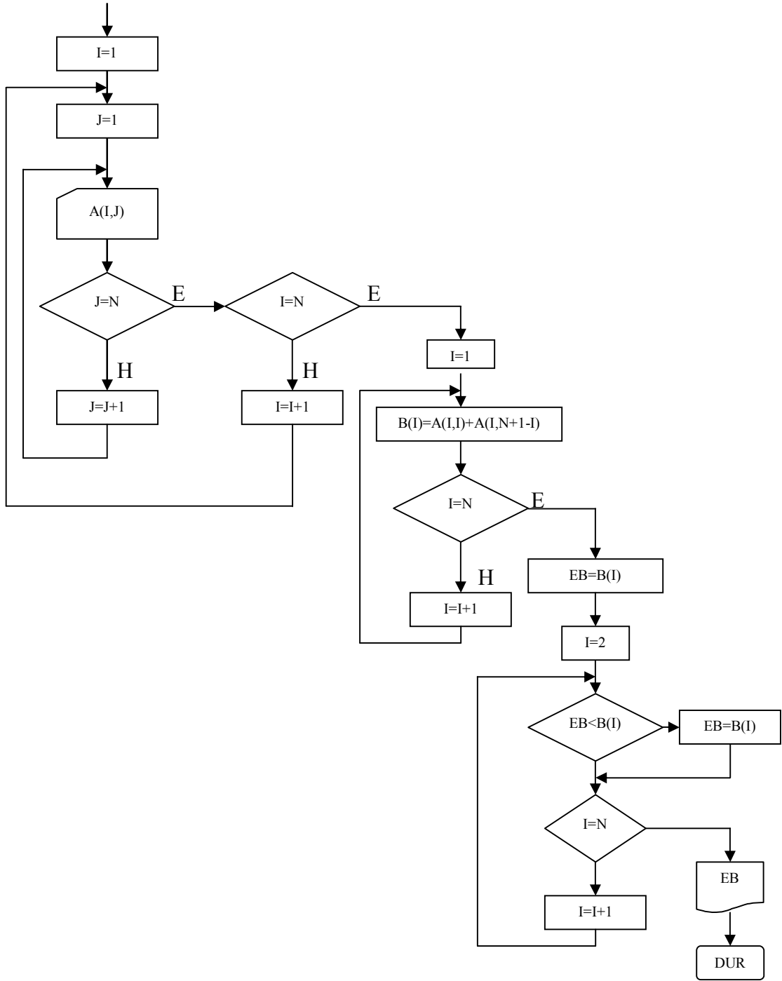
Şekil 4.7.16. N \times N ' lik bir sayı matrisinin esas köşegeni ile yedek köşegeni üzerindeki karşılıklı elemanların çarpımlarını bir diziye yükleyerek bu dizinin en büyük elemanını bulan akış şeması
