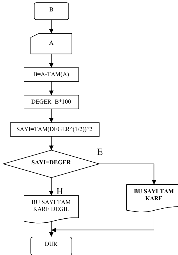
Şekil 4.5.16. Ondalık kısmı iki haneli girilen pozitif bir rasyonel sayının ondalıklı kısmının sayı değerinin bir tam kare olup olmadığını bulan akış şeması.
