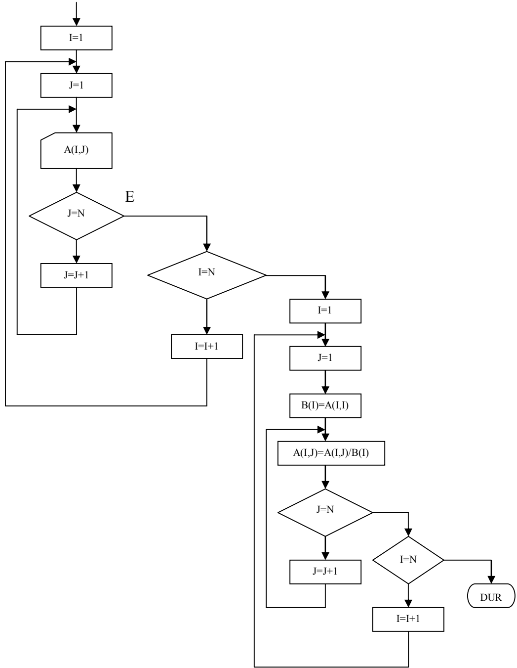
Şekil 4.7.3. NxN' lik bir matrisin esas köşegeni üzerindeki elemanları bir yapan akış şeması
