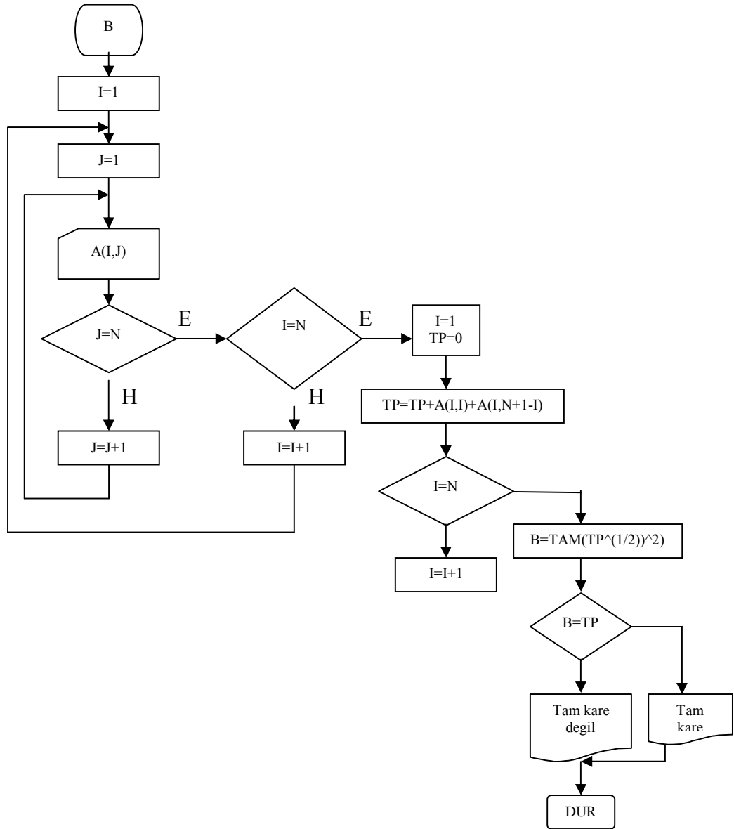
Şekil 4.7.15. NxN' lik bir tamsayı matrisinin esas köşegeni ile yedek köşegeni üzerindeki elemanlarının toplamının bir tam kare sayı olup olmadığını araştıran akış şeması
