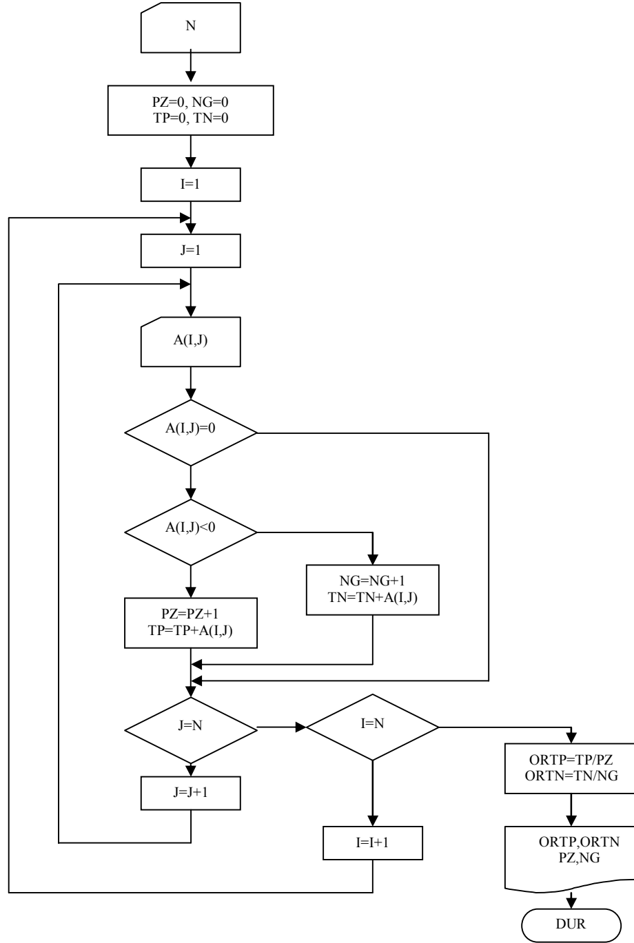
Şekil 4.7.4. NxN' lik bir matrisin negatif ve pozitif elemanlarının sayısını ve ortalamasını bulan akış şeması
